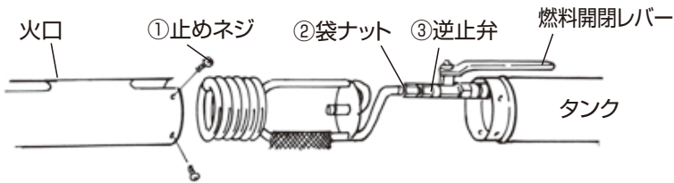
交換用予熱材 KY-12
